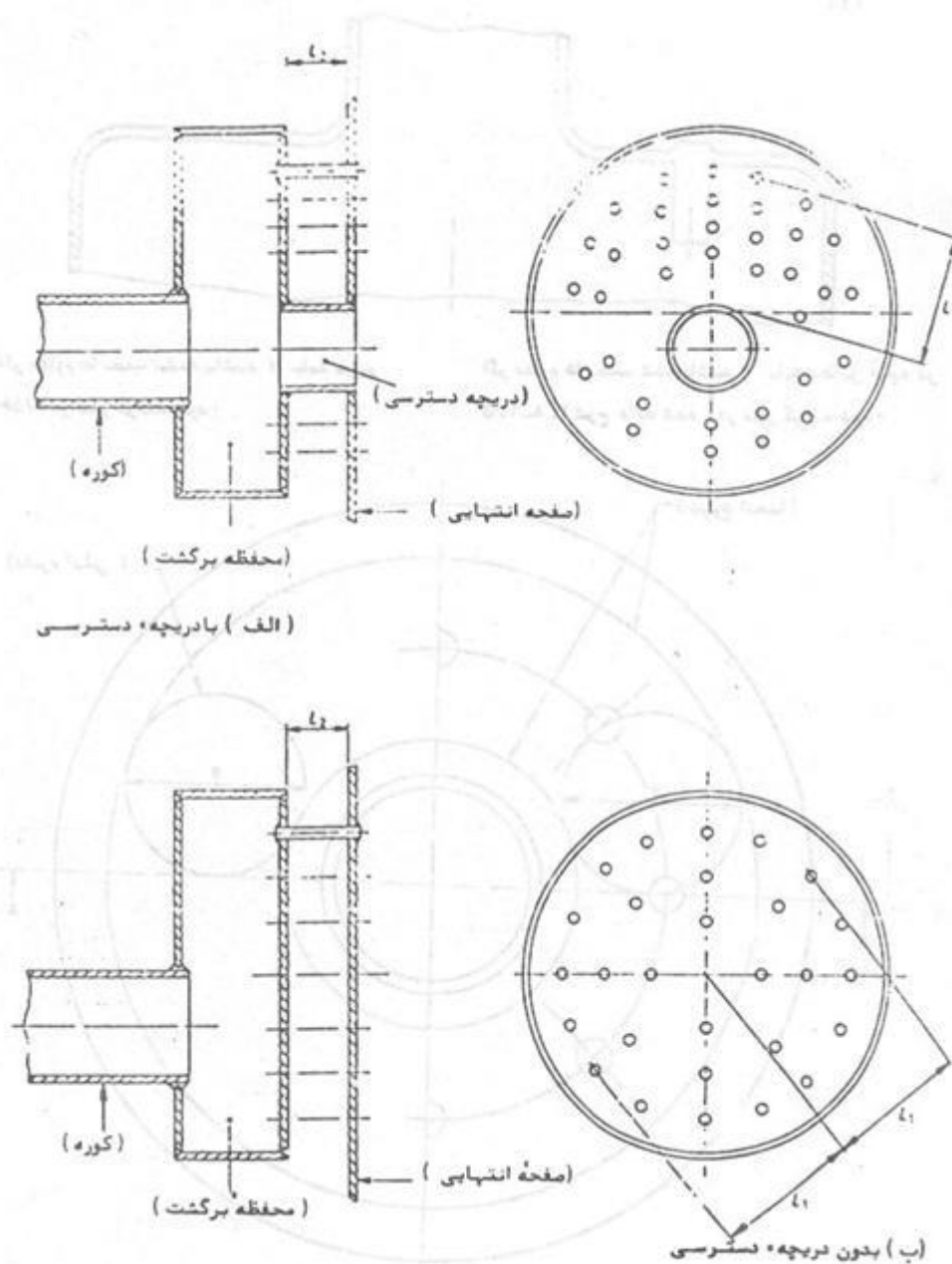
شکل ۵-۸-۱ میل‌های مقاوم برای صفحه + عقبی محفظه های برگشت عقب مربوط
