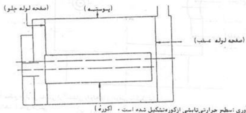
شکل (۴) ۳-۱ دیگ بخار برگشت آتش
