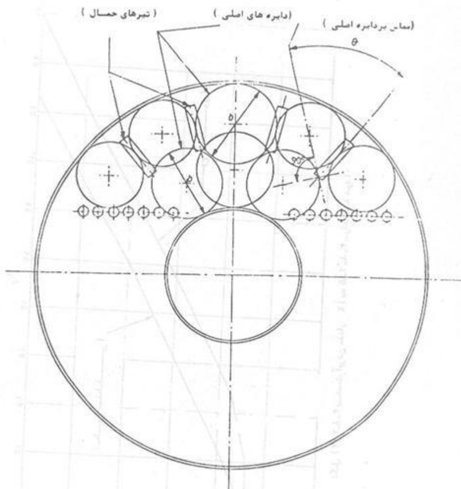
شکل (۲) ۲-۸-۳ نمونه ای از تیر حمال که علاوه بر مماس بودن باید دایره اصلی برخورد نمونه است.
