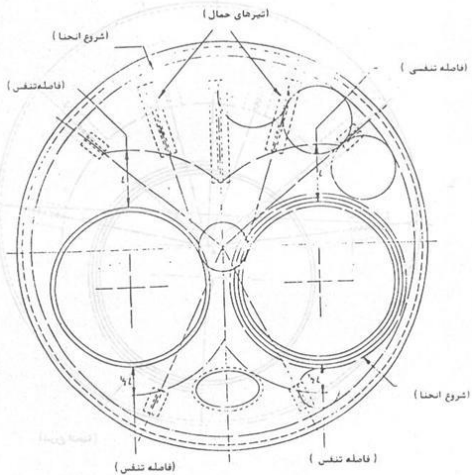
شکل (۳) ۳-۸-۱ ترتیب صفحه انتهایی روی دیگ لانگاساپر
