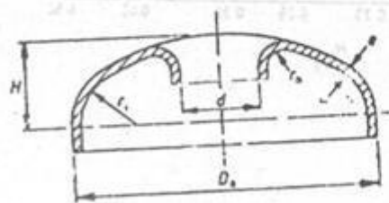
(ج) کله کی باسوراخ آدم رو (نیمه بیضوی یا چنبره کروی)
