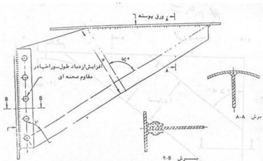
شکل (۲) ۳-۸-۸-۲ جزئیاتی که برای مقاوم های صفحه ای جوش شده و میخی معمول میباشد.
