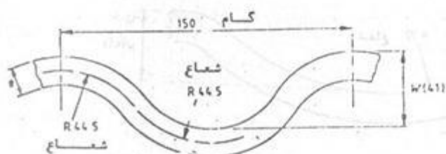
ج - کوره های از نوع فاکس ( با عمق ۴۱ میلیمتر و چین ۱۵۰ میلیمتر )
