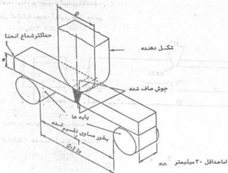
شکل ۵.۴.۶-۱.۳ نحوه برش صفحه آزمایش
