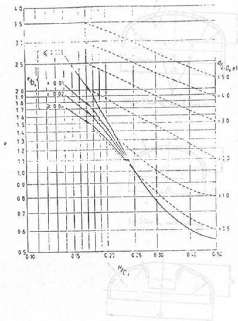
شکل (۲) ۳-۳ ضریب شکل
