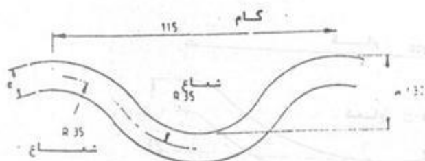
الف - کوره های ازبوع فاکس و با عمق ۳۰ میلیمتر و چین ۱۱۵ میلیمتر )
